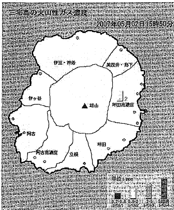
図 三宅島火山性ガス濃度 引用) 三宅村ホームページ( http://www.miyakemura.com )
